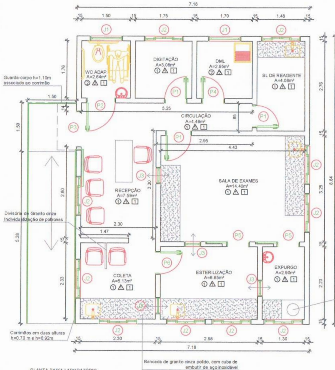
PLANTA BAIXA LABORATÓRIO ESC: 1/50
