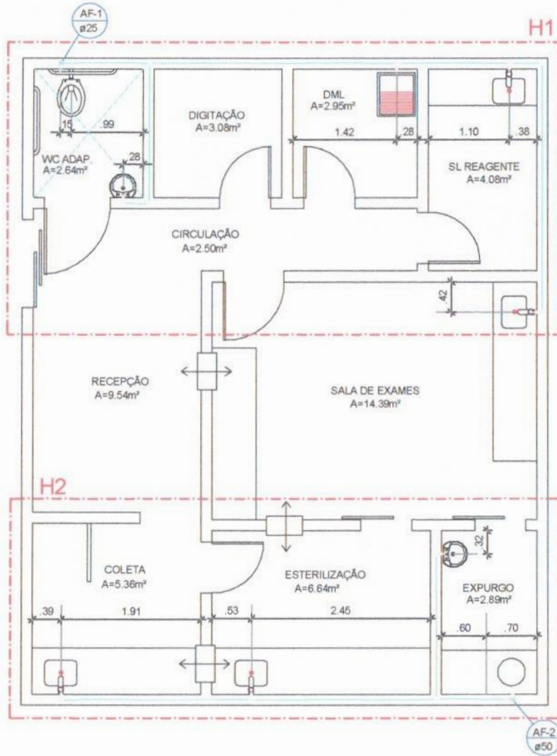
PLANTA BAIXA LABORATÓRIO - INST. HIDRÁULICAS ESC: 1/50
