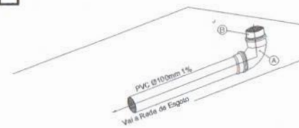
DETALHE EXECUTIVO DE ESGOTO RAMAL DRENO LAVADORA COM BARREIRA
