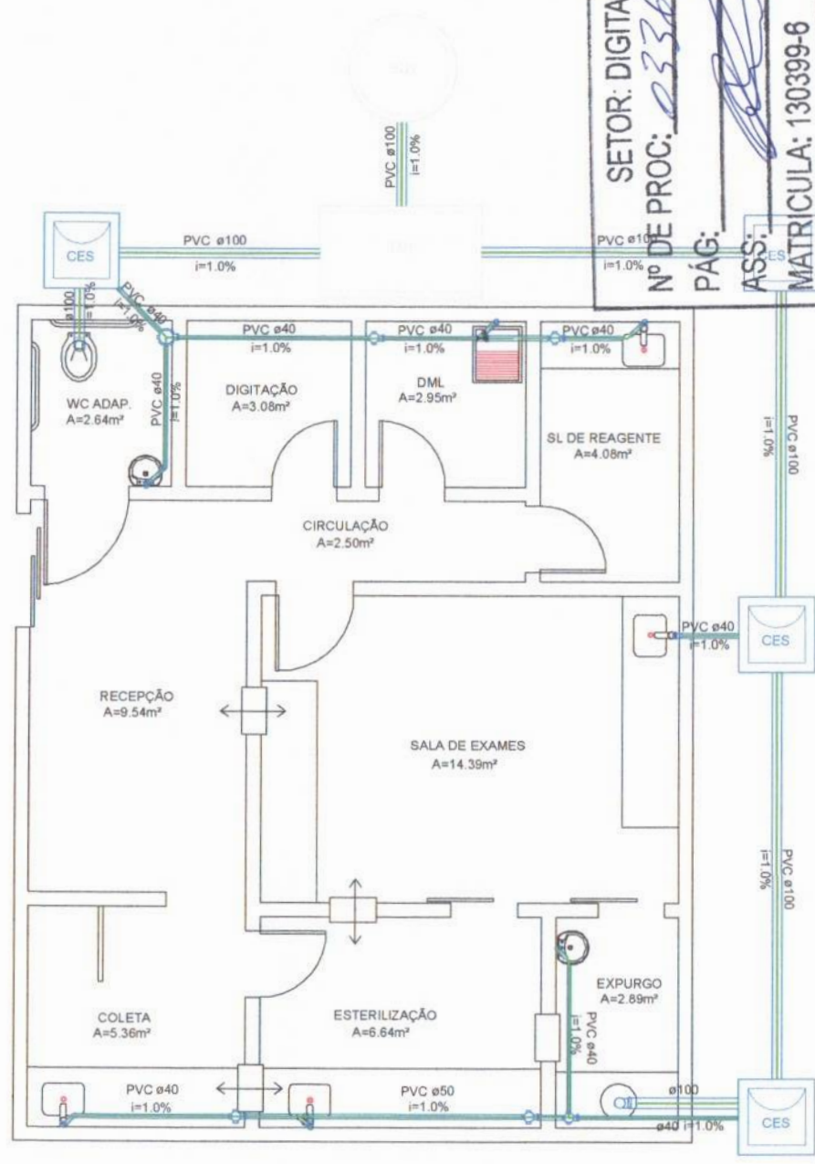
PLANTA BAIXA LABORATÓRIO - INST. SANITÁRIAS ESC: 1/50
