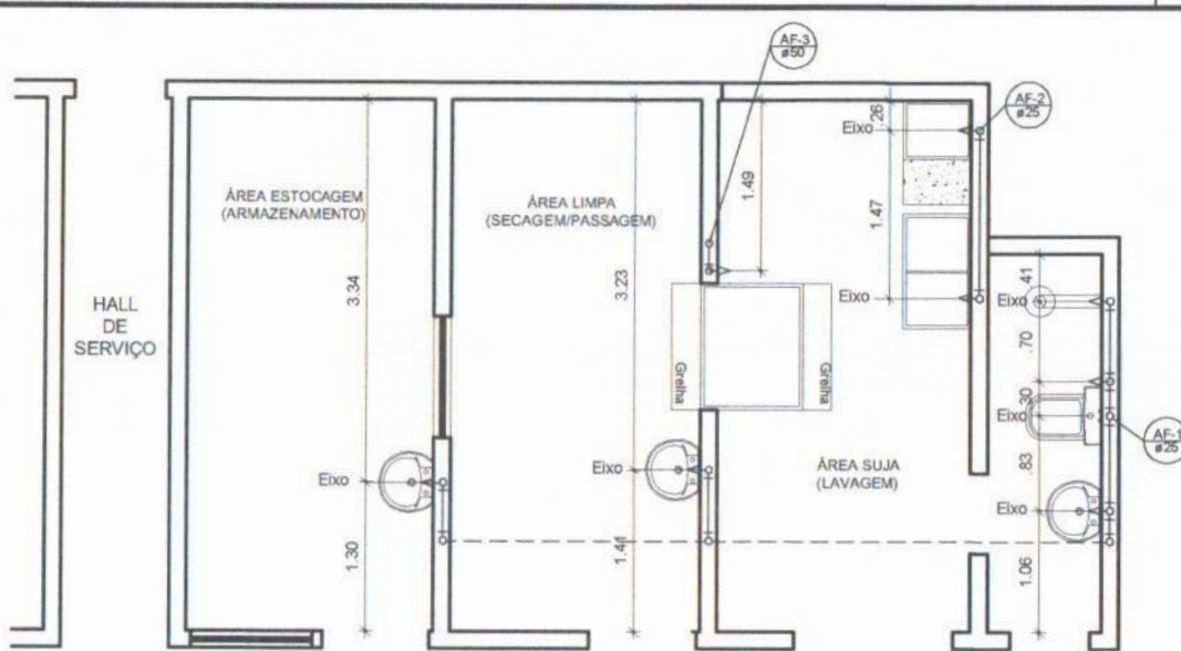
PLANTA BAIXA - PONTOS HIDRÁULICOS ESCALA 1/50
