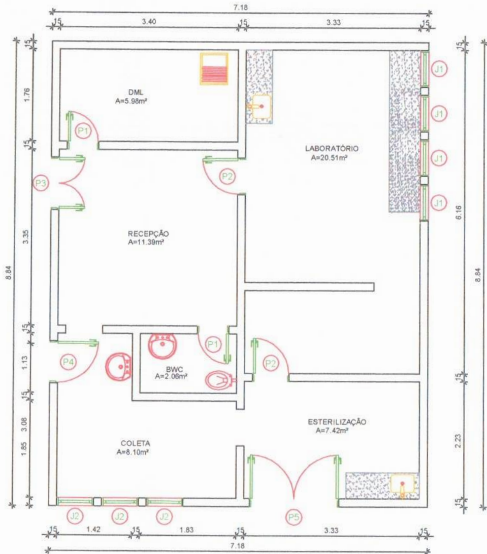
PLANTA BAIXA EXISTENTE ESC: 1/50
