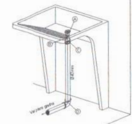
DETALHE EXECUTIVO DE ESGOTO RAMAL TANQUE SEM SIFÃO
