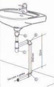
DETALHE EXECUTIVO DE ESGOTO RAMAL LAVATÓRIO COM SIFÃO
