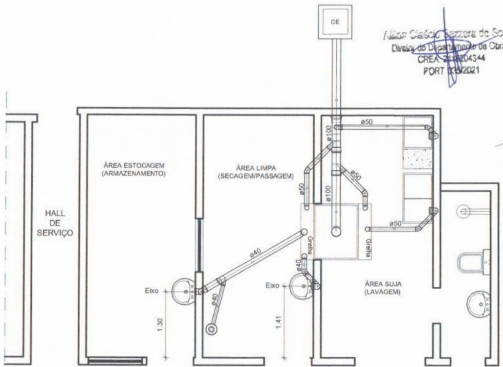
PLANTA BAIXA - PONTOS SANITÁRIOS ESCALA 1/50
